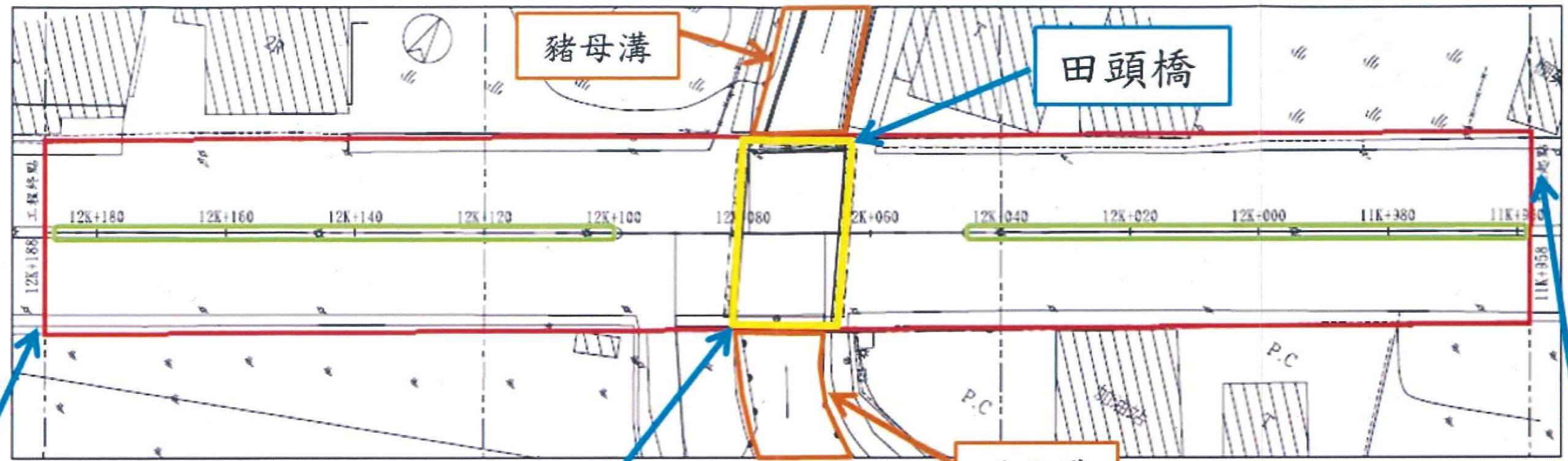
路權圖
